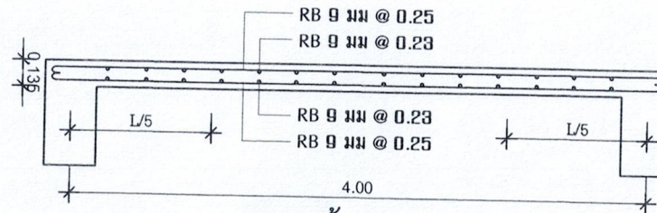
ขยายพื้น S1
