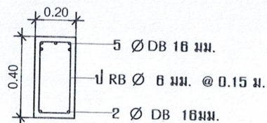
ขยายคาน CB
