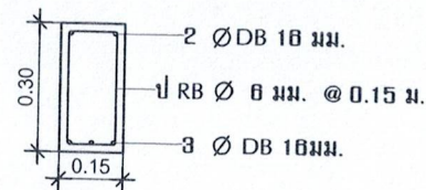
รูปตัด 2
