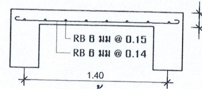
ขยายพื้น S
