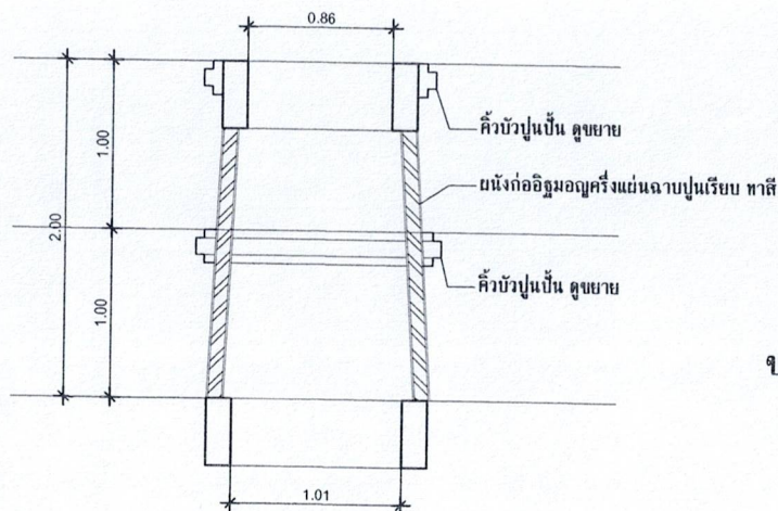
รูปตัดปล่องคว้น
