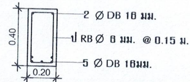
รูปตัด 4
