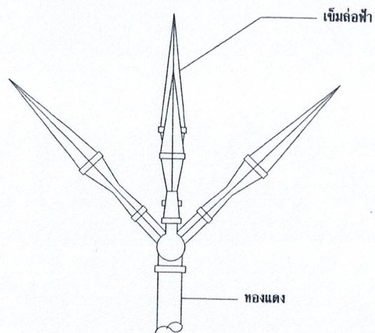
แบบขยายสายล่อปลา
