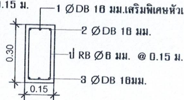
รูปตัด 1
