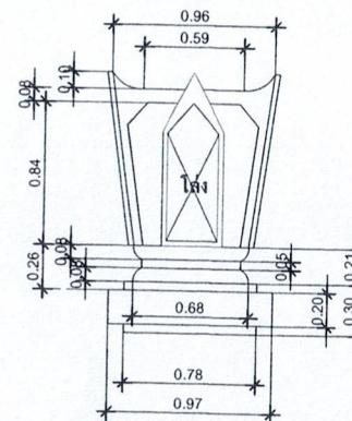
ขยายครอบปล่อง
