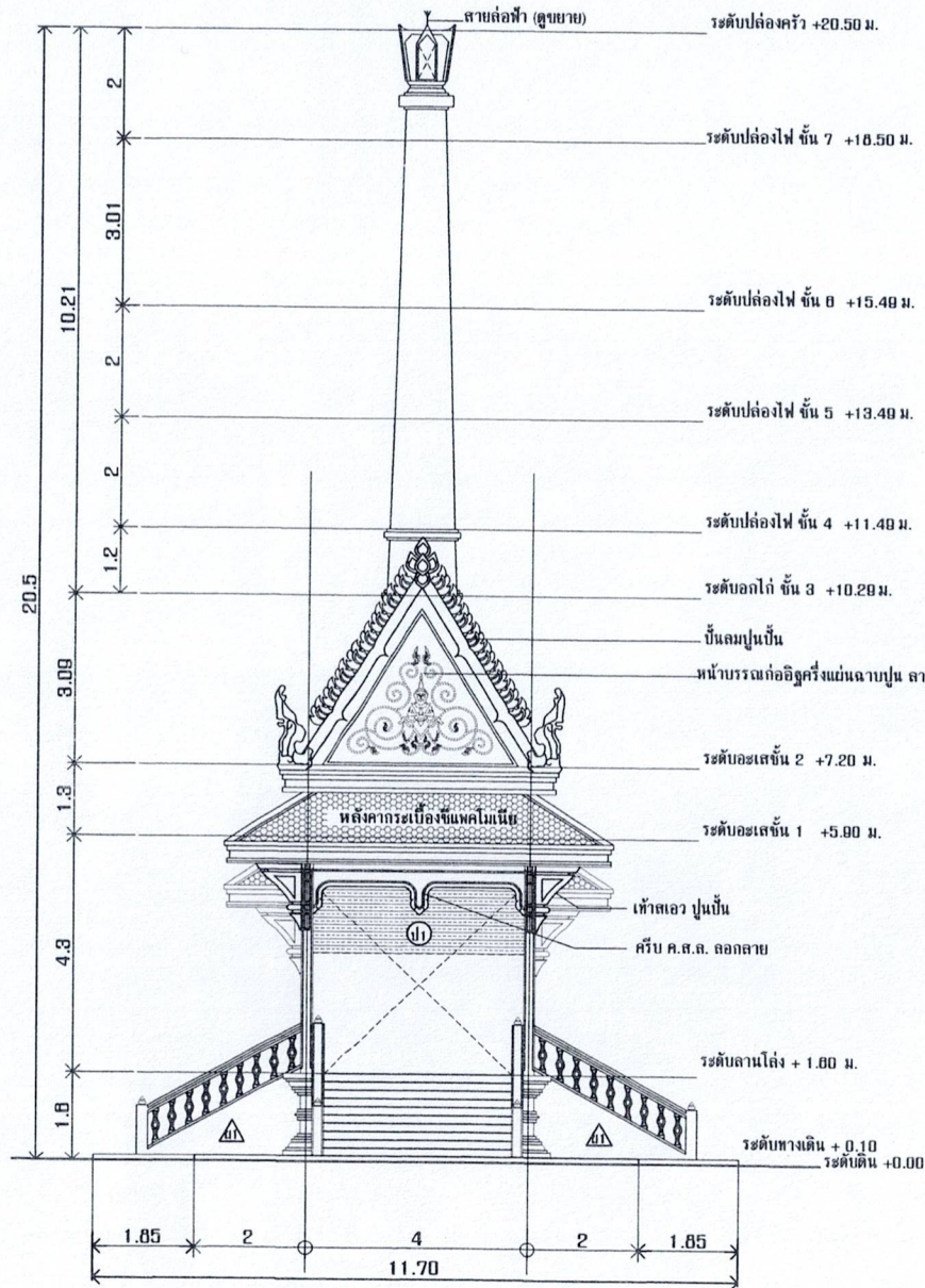
รูปด้านข้าง 2 มาตราส่วน 1:150
