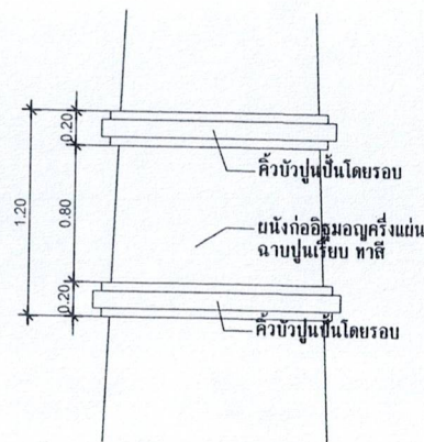
ขยายปล่องคว้น
