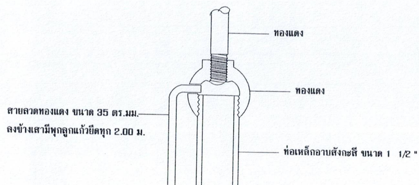
ขยายสายล่อปลา (จุด ก)
