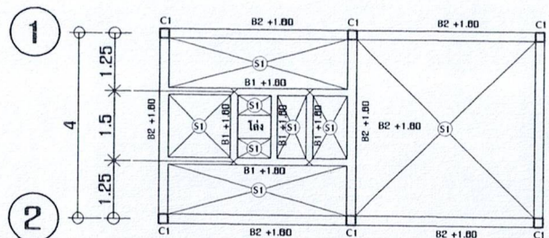
โครงสร้างคาน พื้น มาตราส่วน 1:150
