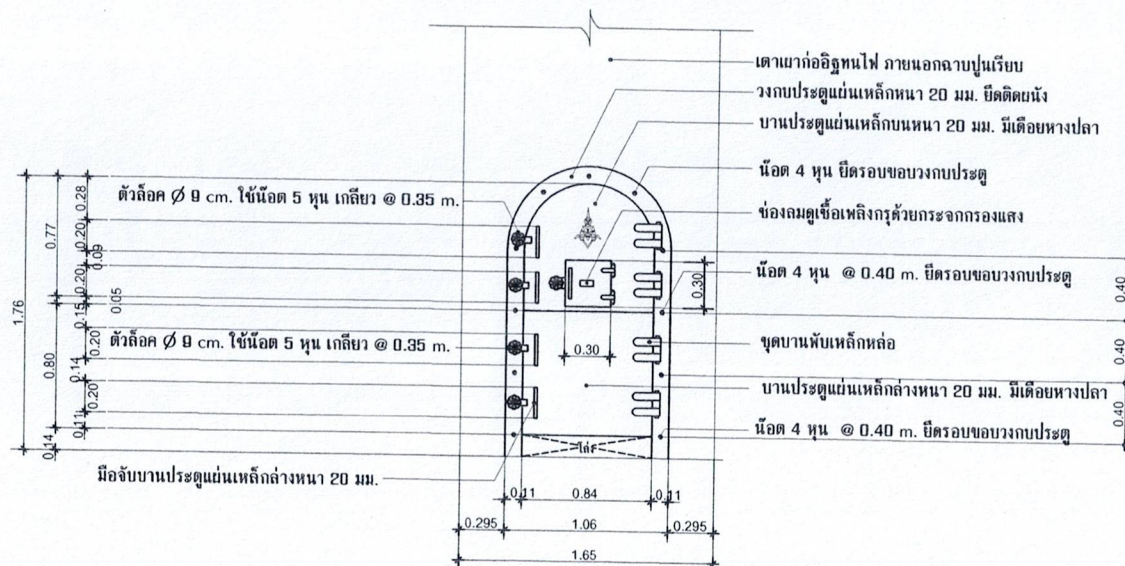
รูป หน้าเตาเผา มาตราส่วน 1:50
