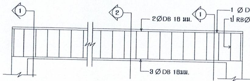
ขยายคาน GB1,B1
