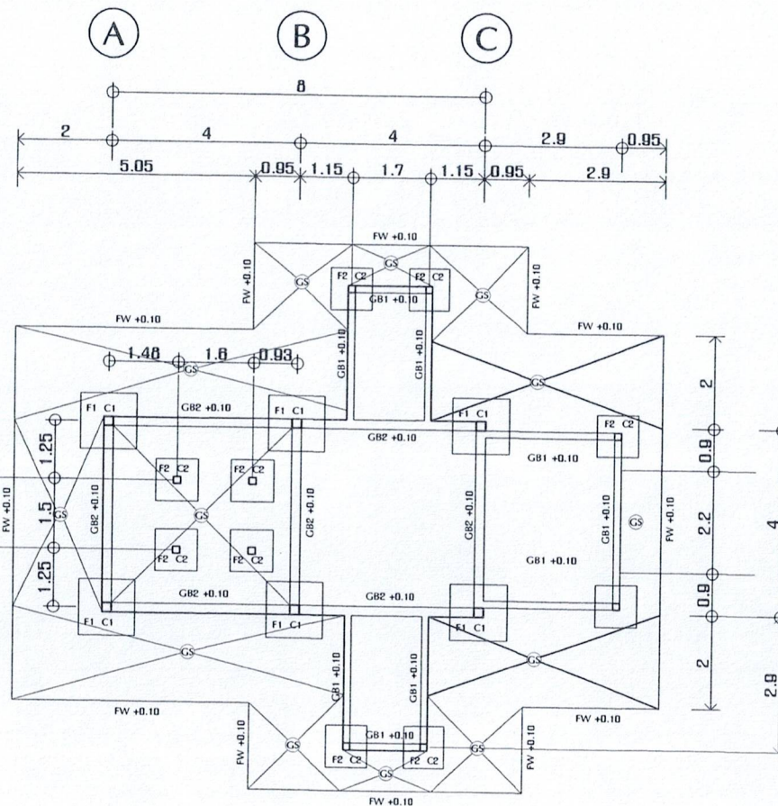
โครงสร้างฐานราก คานคอดิน มาตราส่วน 1:150
