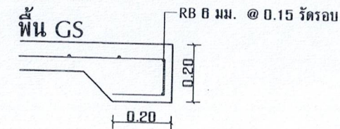
ขยายคอรืงราก FW
