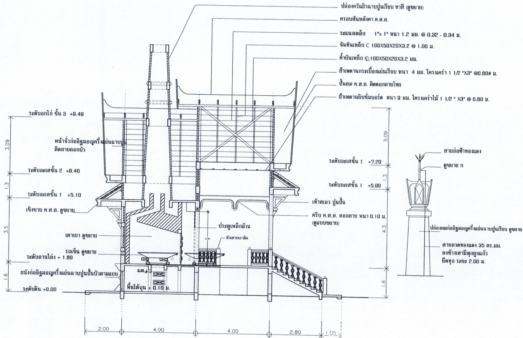
รูปตัดแนวน B - B มาตราส่วน 1:125
