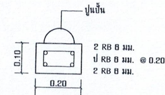
ขยายราบบันได คสล.
