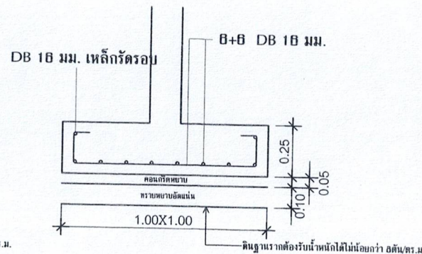
ขยายฐานราก F2
