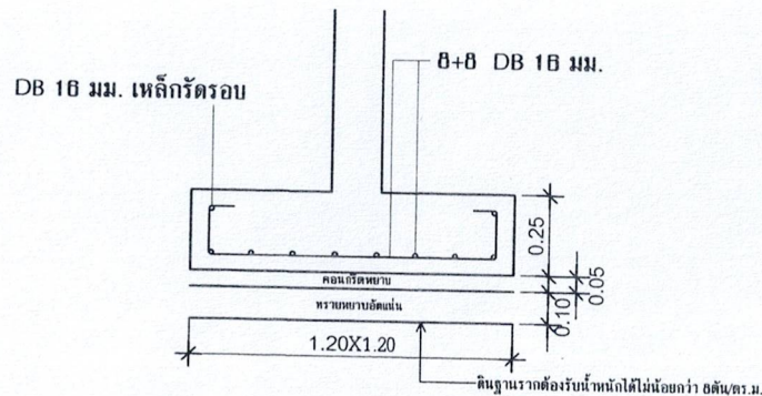
ขยายฐานราก F1
