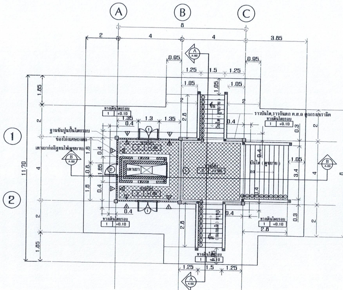
แปลนพื้นที่ชั้นล่าง มาตราส่วน 1:150
