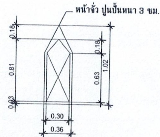
ขยายหน้าจั่วครอบปล่อง
