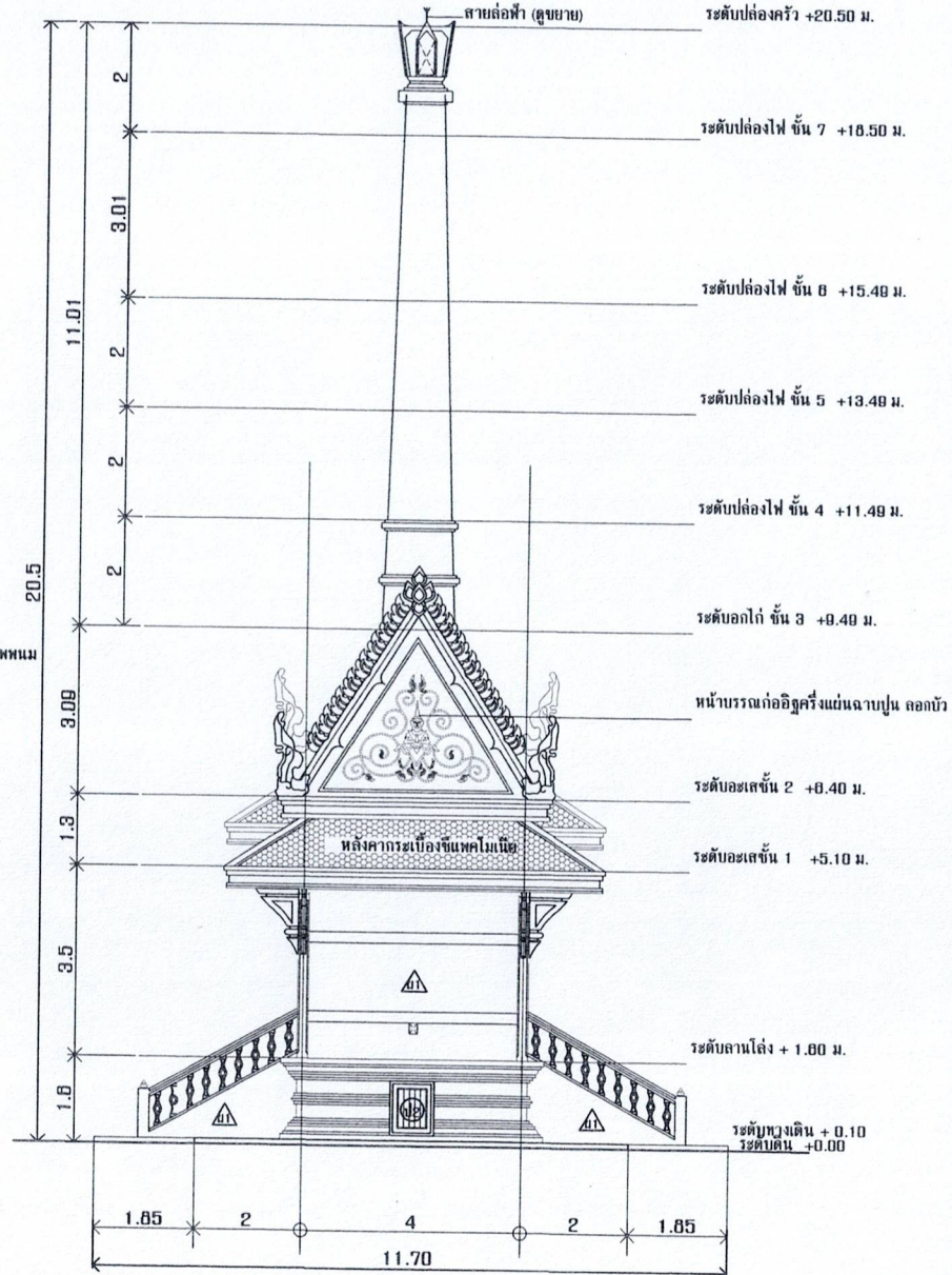
รูปด้านข้าง 4 มาตราส่วน 1:150
