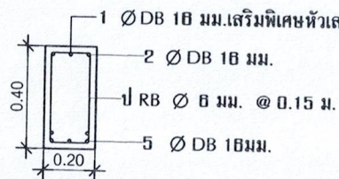
รูปตัด 3
