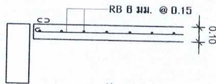
ขยายพื้น GS
