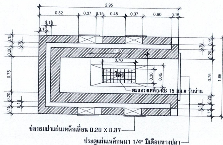
แปลนเตาเผา มาตราส่วน 1:50
