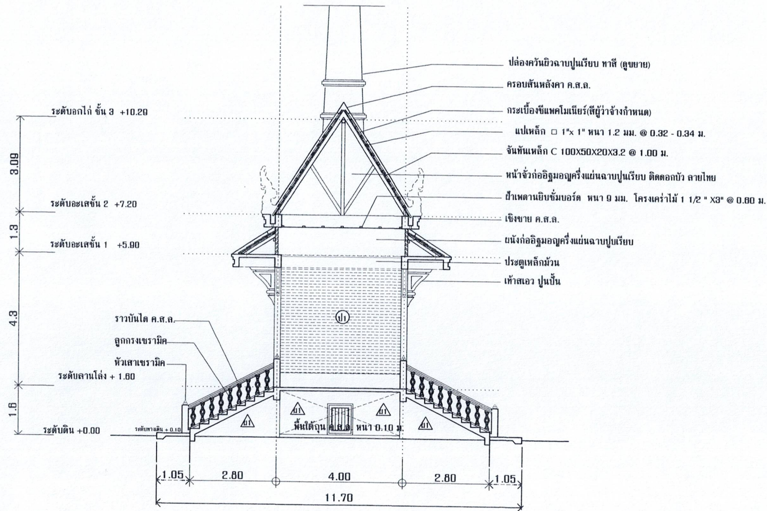
รูปตัด A - A มาตราส่วน 1:125
