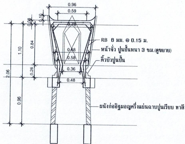
รูปตัดครอบปล่อง
