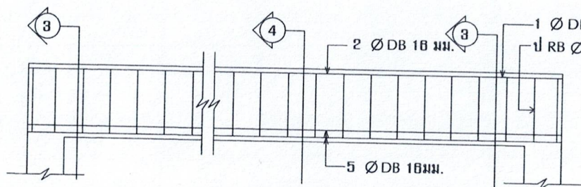
ขยายคาน GB2,B2
