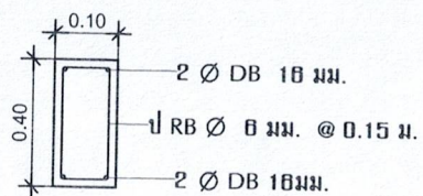
ขยายคาน B3
