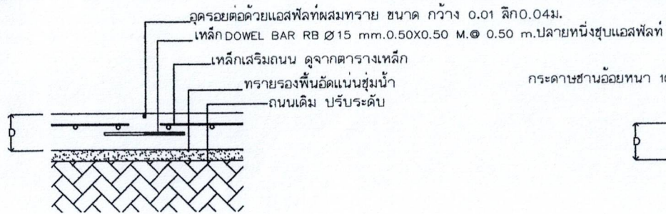
CONTRACTION JOINT ทุกกระยะ = ( 10.00 ม )
