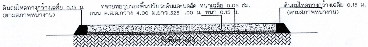
แปลนแสดงรูปตัด
