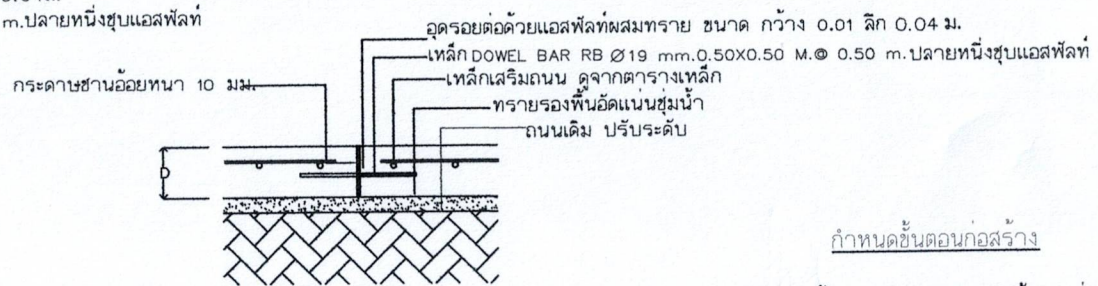
EXPANSION JOINT ทุกกระยะ = ( 40.00 ม )
